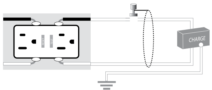
LE COURANT i_3 EST DEVENU > 5 mA LE DISJONCTEUR A DÉCLENCHÉ. LE COURANT NE CIRCULE PLUS. LE DÉFAUT D'ISOLEMENT EST TOUJOURS PRÉSENT.
