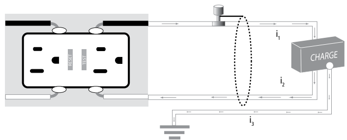
IL Y A UN DÉFAUT D'ISOLEMENT. UNE CERTAINE QUANTITÉ DE COURANT ( i_3 ) CIRCULE AILLEURS QUE DANS LE CIRCUIT NORMAL ; i_1 = i_2 + i_3 .
